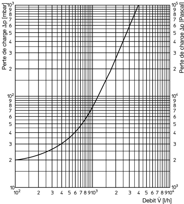
Diagramme de débit «Regumat RTA-180» DN 32
