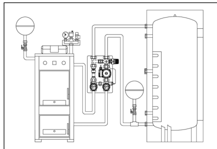
Abb. 5 Einbindung eines „Regumaten“ zwischen Feststoffkessel und Pufferspeicher
