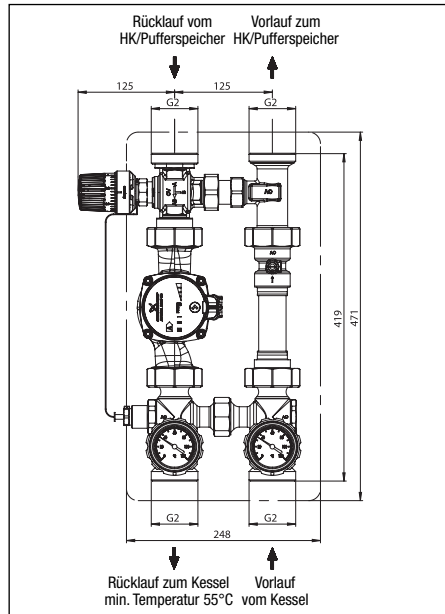
Abb. 4.6 „Regumat RTA-180“ DN32 mit Standardisolation Vorlauf auf der rechten Seite Kessel ist unterhalb der Station angeordnet
