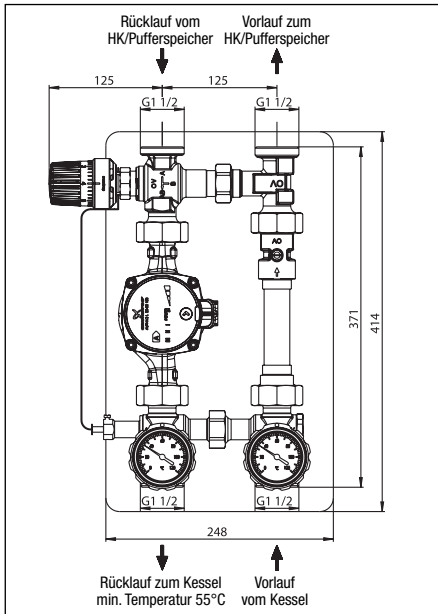
Abb. 4.4 „Regumat RTA-180“ DN25 mit Universalisolation Vorlauf auf der rechten Seite Kessel ist unterhalb der Station angeordnet
