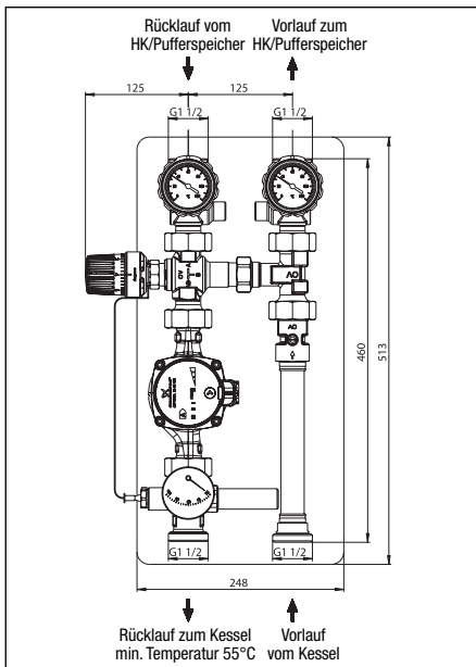
Abb. 4.5 „Regumat RTA-180“ DN25 mit Standardisolation Vorlauf auf der rechten Seite Kessel ist unterhalb der Station angeordnet
