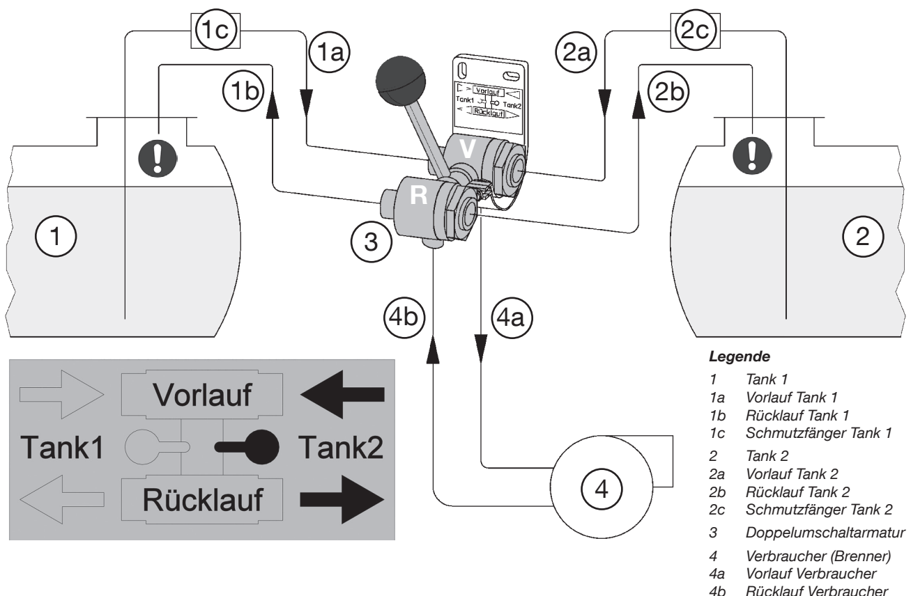
Anschluss-Skizze Doppelumschaltarmatur
