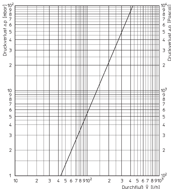
Durchflussdiagramm, Strömungswiderstand im Vorlauf
