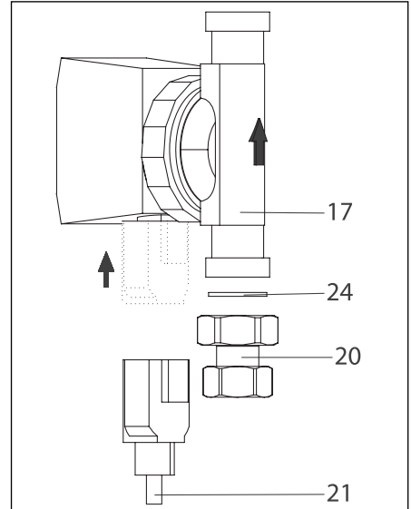
Abb. 6.2 Pumpenausrichtung
