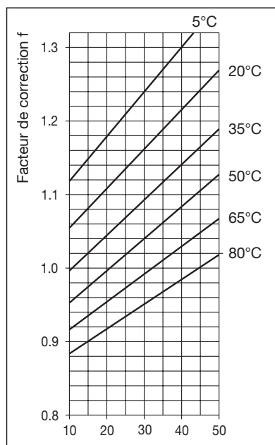
% masse éthylèneglycol
