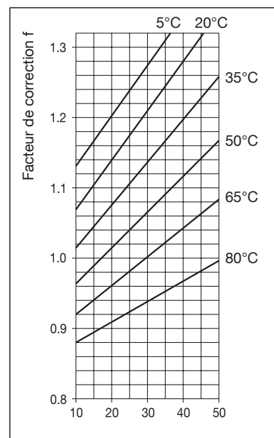
% masse propylèneglycol
