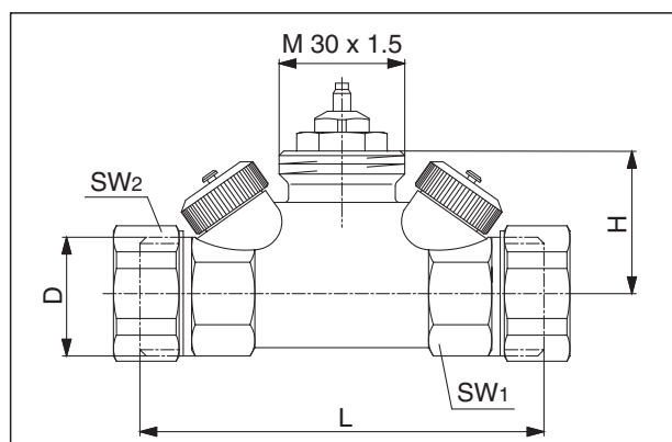
Encombrements « Hycoco ETZ/HTZ » avec filetage femelle
