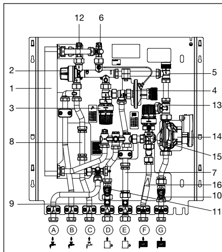
Fig. 5.2 Installazione con circuito di riscaldamento misto
