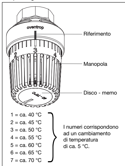
Fig. 8.3 Regolazione temperatura acqua sanitaria
