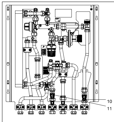
Fig. 8.1 Posizione d'installazione filtro
