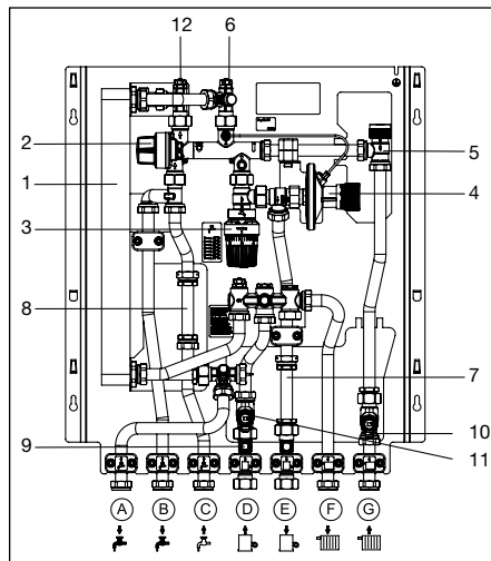
Fig. 5.1 Conception avec circuit de chauffage direct
