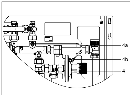
Fig. 8.2 Purge
