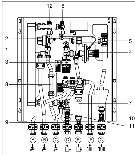
Abb. 5.1 Aufbau mit direktem Heizkreis
