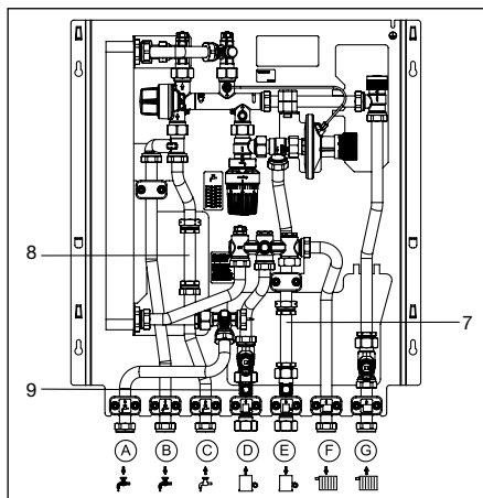
Abb. 6.1 Einbau Kaltwasser- und Wärmezähler
