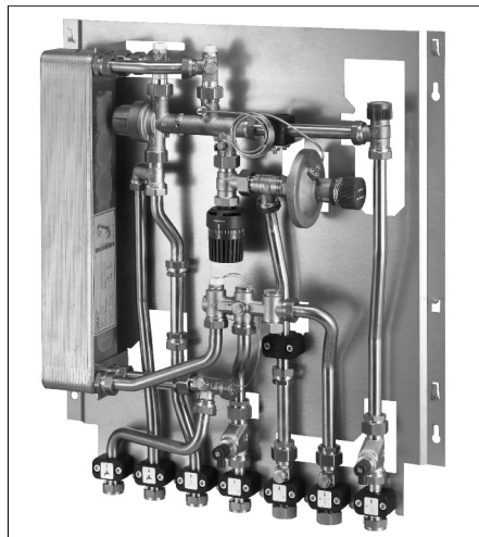
Abb. 1.1 „Regudis W-HTF“ Wohnungsstation
