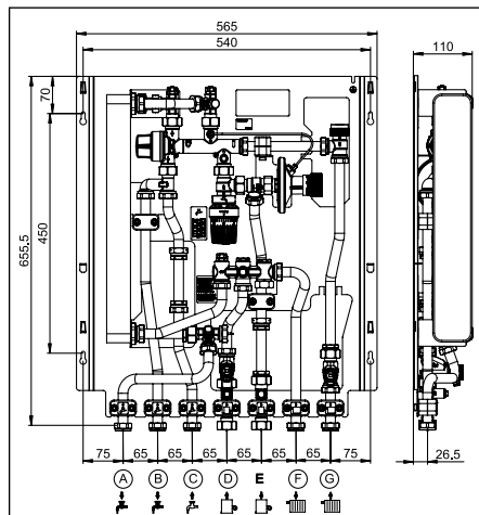
Fig. 4.2 Dimensioni con circuito di riscaldamento diretto
