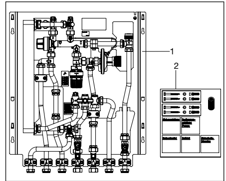
Abb. 3.1 Lieferumfang
