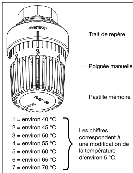
Fig. 8.3 Réglage de la température d'eau chaude sanitaire
