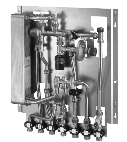
Fig. 1.1 Station d'appartement «Regudis W-HTF»
