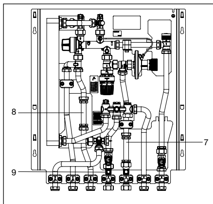
Fig. 6.1 Installazione contatore acqua fredda e contacalorie
