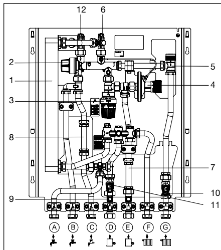
Fig 5.1 Struttura con circuito di riscaldamento diretto
