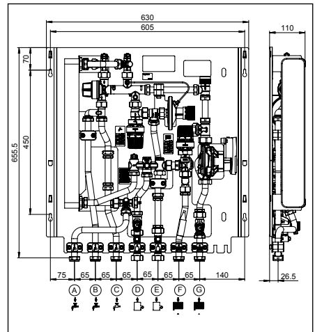
Abb. 4.4 Abmessungen mit gemischtem Heizkreis
