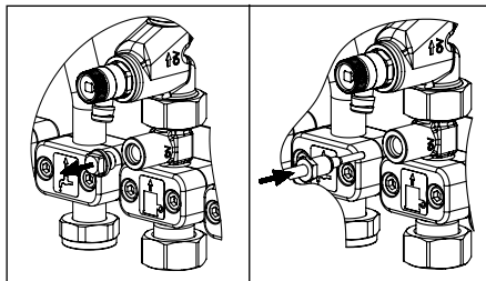
Abb. 6.2 Einbau Fühler für Wärmezähler
