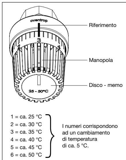
Fig. 8.4 Regolazione temperatura mandata riscaldamento
