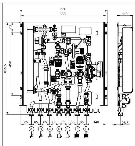
Fig. 4.4 Dimensioni con circuito di riscaldamento miscelato
