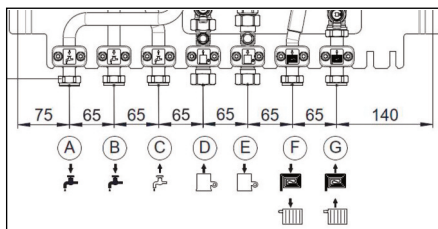
Abb. 4.3 Anschlussmaße
