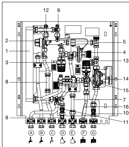
Fig. 5.2 Conception avec circuit de chauffage mélangé
