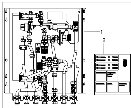
Fig. 3.1 Componenti inclusi nella fornitura
