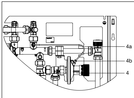
Illustr. 8.2 Bleeding
