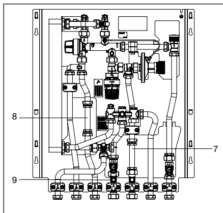
Fig. 6.1 Montage du compteur d'eau froide et du compteur de calories
