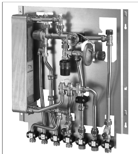
Fig. 1.1 Modulo satellite per unità abitativa “Regudis W-HTF”
