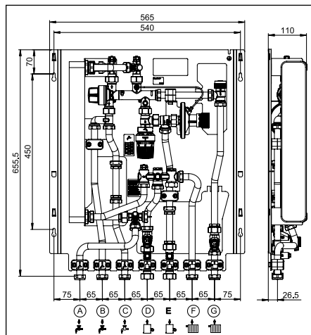
Fig. 4.2 Encombrements avec circuit de chauffage direct
