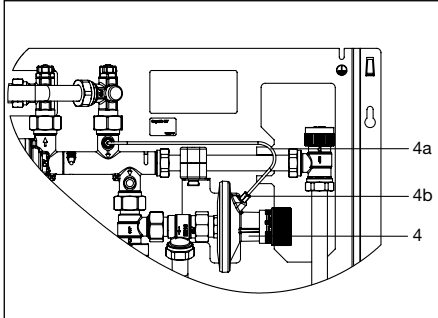
Abb. 8.2 Entlüftung
