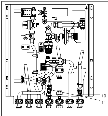
Fig. 8.1 Position de montage des filtres
