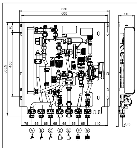
Fig. 4.4 Encombrements avec circuit de chauffage mélangé
