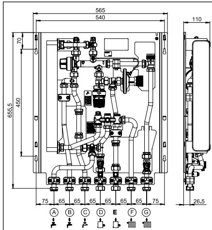
Abb. 4.2 Abmessungen mit direktem Heizkreis
