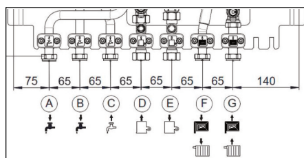
Fig. 4.3 Dimensioni collegamenti
