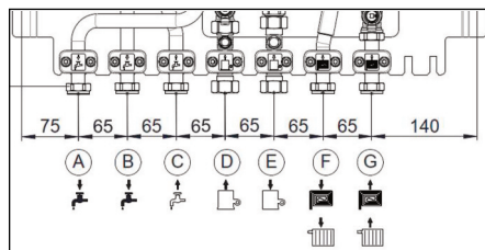
Fig. 4.3 Cotes de raccordement
