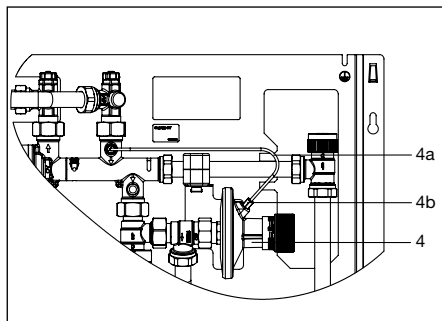
Fig 8.2 Sfiato
