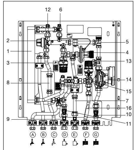
Abb. 5.2 Aufbau mit gemischtem Heizkreis
