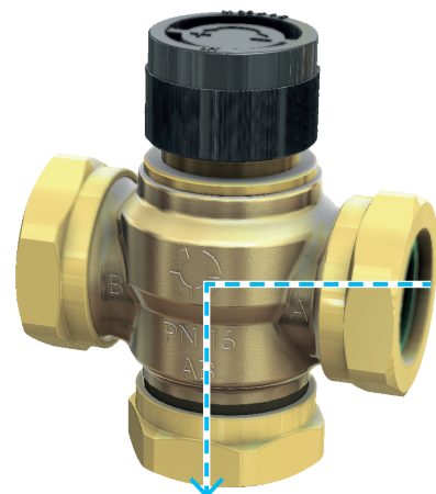
Abb. 2: Durchfluss A-AB
