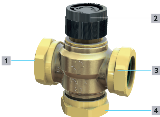
Abb. 1: Aufbau Dreiwegeventil
