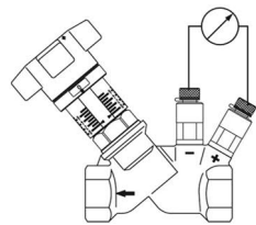
Mesure de la pression différentielle via le robinet HydroControl MTR. Permet de mesurer le débit sur la base de la pression différentielle via l'orifice de mesure HydroControl MTR et de la valeur kv enregistrée dans l'ordinateur de mesure OV-DMC 3.
