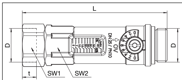
Encombrements
