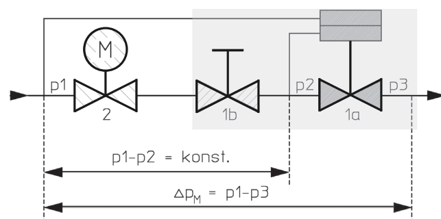
Рис. 3: Принцип функционирования «Cocon QTZ», PN25
