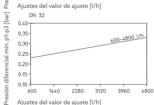
Fig. 13: Presiones diferenciales mínimas
