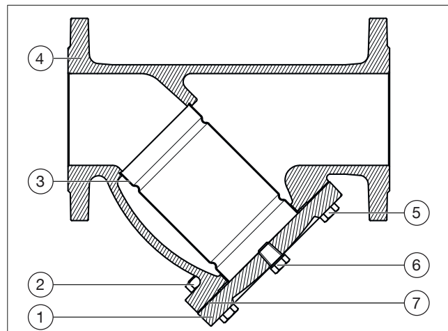
Abb. 1: Schmutzfänger Aufbau
