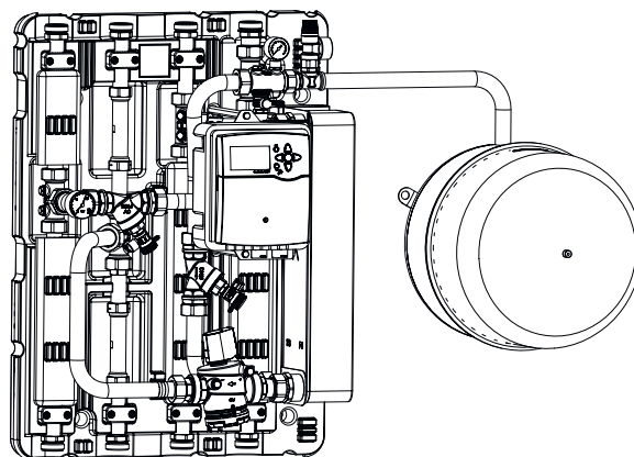
Fig. 40: Vase d'expansion à membrane monté
