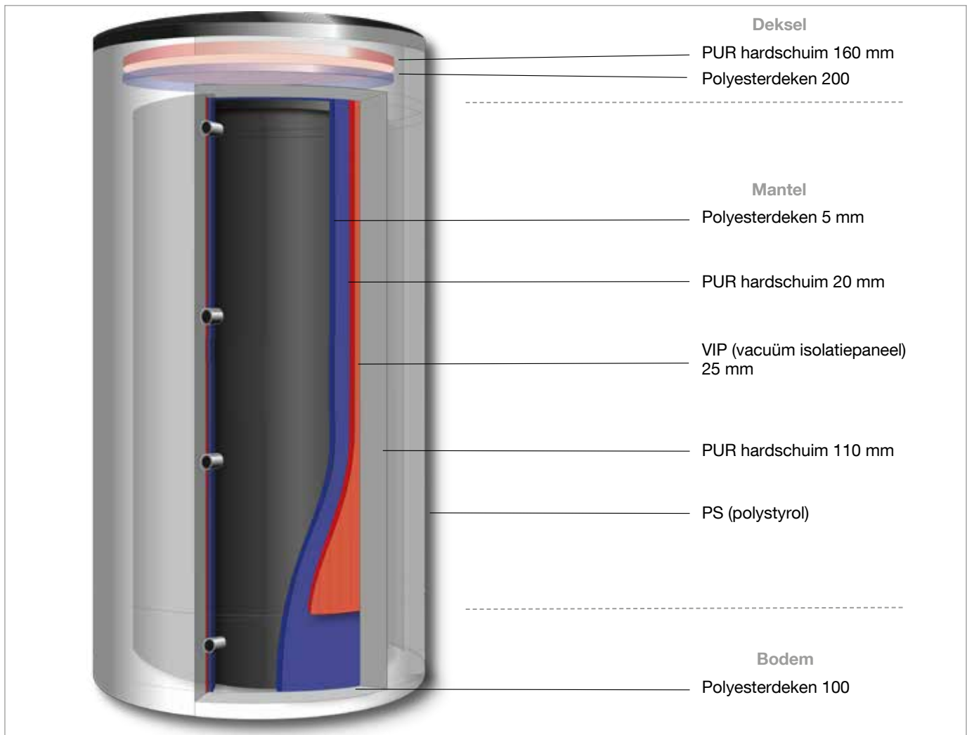
Opbouw van de isolatie van de Regucor WHS, model 500, energie-efficiëntieklasse
