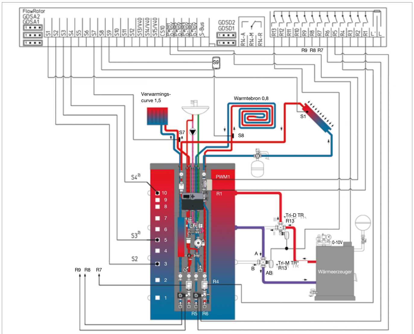
Regucor WHS met twee gekoppelde weersafhankelijke gestuurde verwarmingsgroepen en een conventionele warmtebron met warmtetoevoer en omschakeling tussen de bufferlagen.
