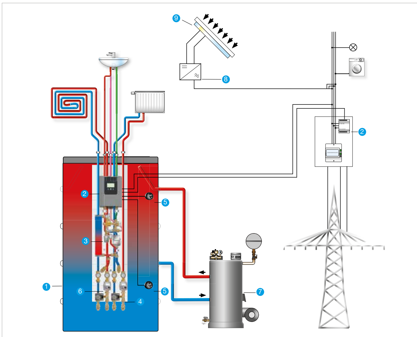
Regucor WHP systeem gecombineerd met conventionele warmtebronnen
