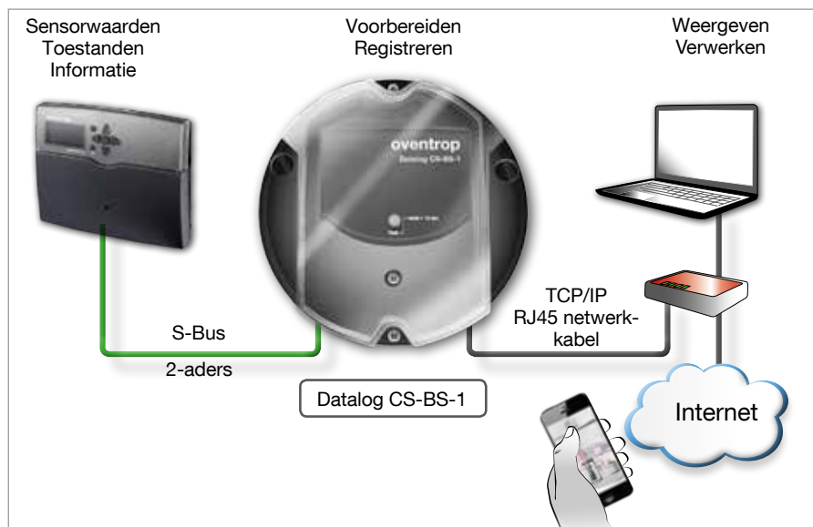
Systeem op basis van de DynaTemp CS-BS als oplossing en datalogger
