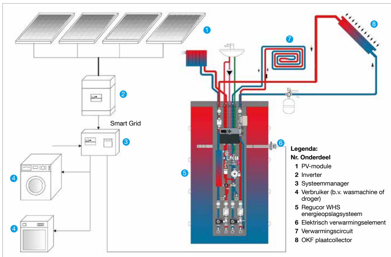
PV/Smart Grid systeem (voorbeeld)
