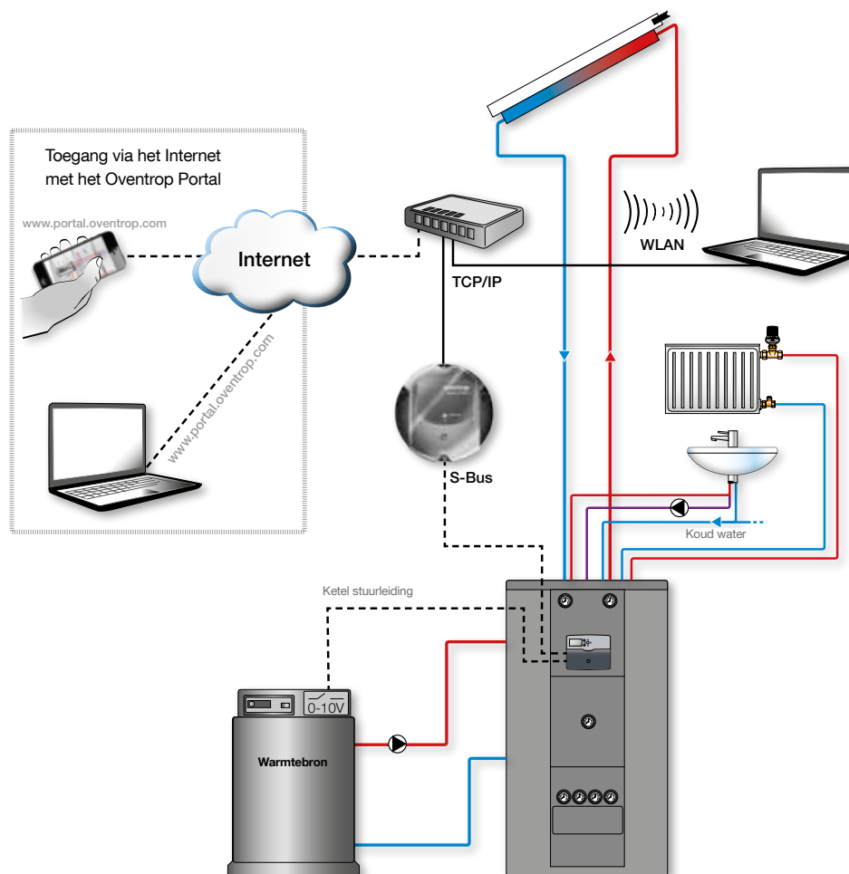
Regucor WHS energieopslagsysteem voor zonneverwarming, tapwater en verwarming
