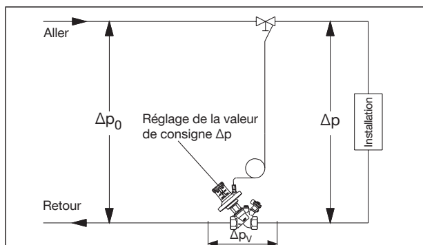
Schéma d'installation
