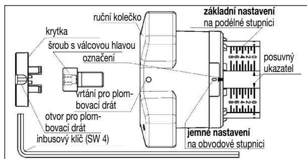
Obr. 7.1 Přednastavení
