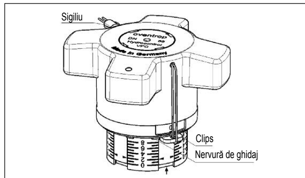
Fig. 7.2 Blocarea rozetei manuale
