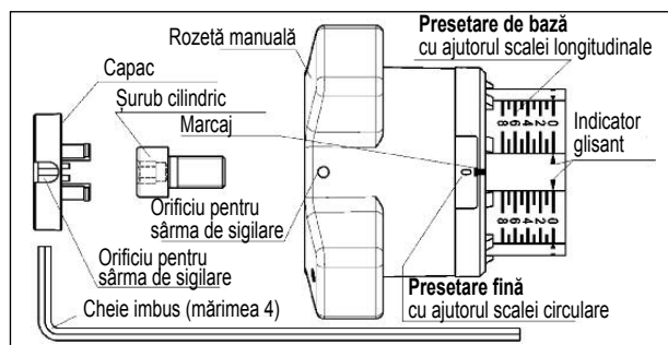
Fig. 7.1 Presetarea
