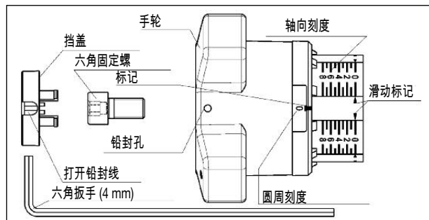
图 7.1 预设
