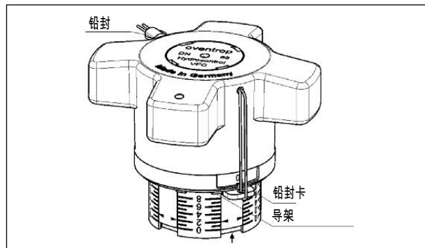
图7.2 手轮的锁定
