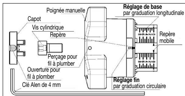
Fig. 7.1 Pré-réglage
