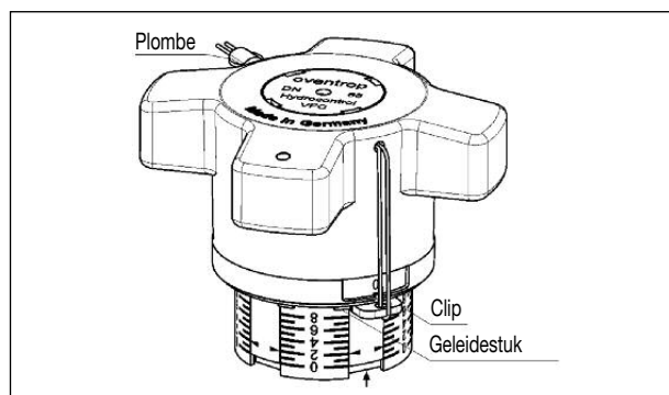
Afb. 7.2 Blockierung van de handregelknop
