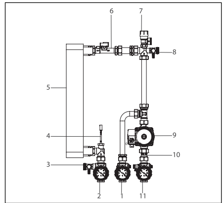
Abb. 7: Sekundärkreislauf mit Asynchron-Zirkulationspumpe
