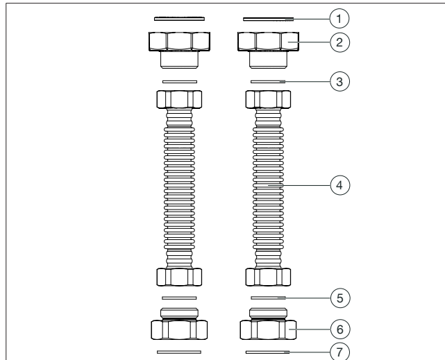
Abb. 35: Aufbau Verbindungsset
