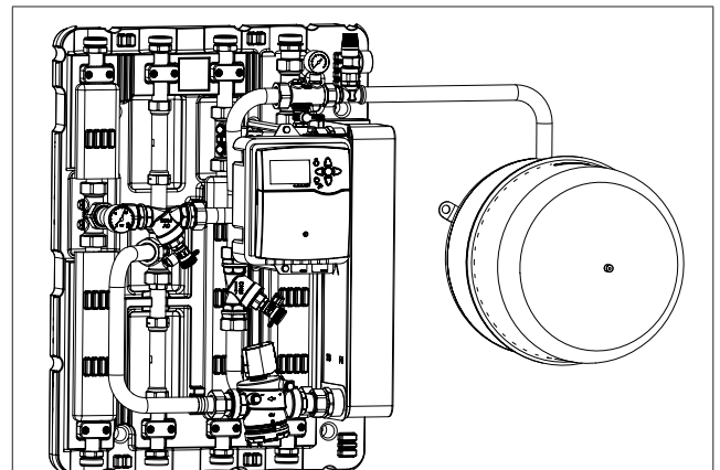
Abb. 39: Membranausdehnungsgefäß montiert
