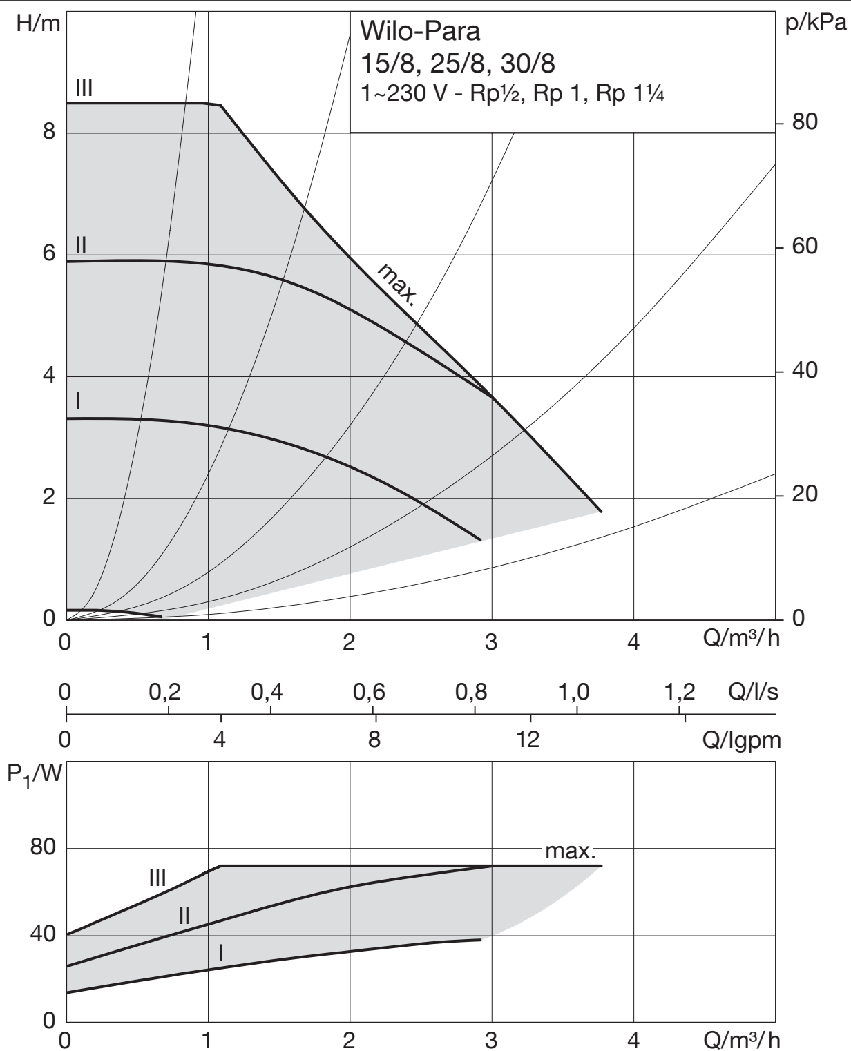
Abb. 60: Pumpenkennlinie Drehzahl konstant
