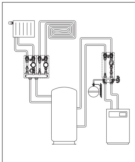
Abb. 5.2 Systembild Heizkreis-Anschlussgruppe
