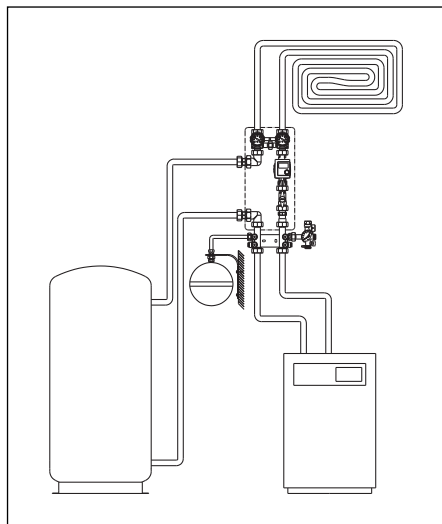
Abb. 5.1 Systembild Pufferspeicher-Anschlussgruppe
