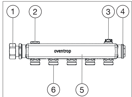
Abb. 1: Aufbau
