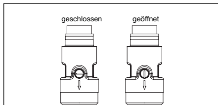
Abb. 21 Schwerkraftbremse
