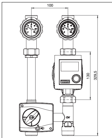
Abb. 23 Abmaße „Regumat M3-130“ DN20
