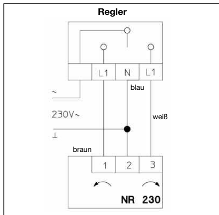
Abb. 22 Regler
