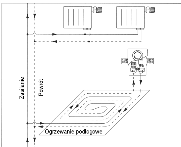
Szkic zabudowy modułu do regulacji temperatury pomieszczenia i ograniczania temperatury w rurze instalacji
