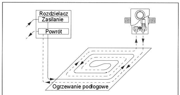
Szkic zabudowy modułu do regulacji temperatury pomieszczenia
