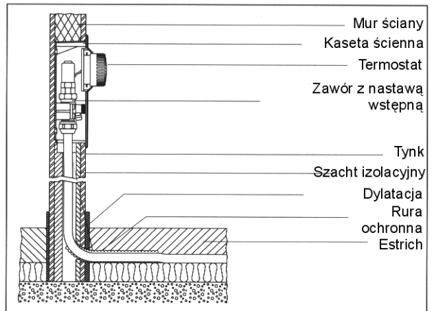
"Unibox E T", głębokość zabudowy 57 mm
