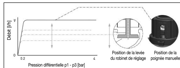
Fig. 7 Courbe de fonctionnement du débit pour différents pré-réglages
