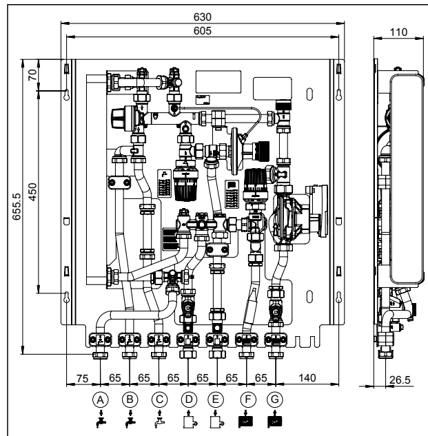
Dimensiuni cu circuit cu temperatură variabilă
