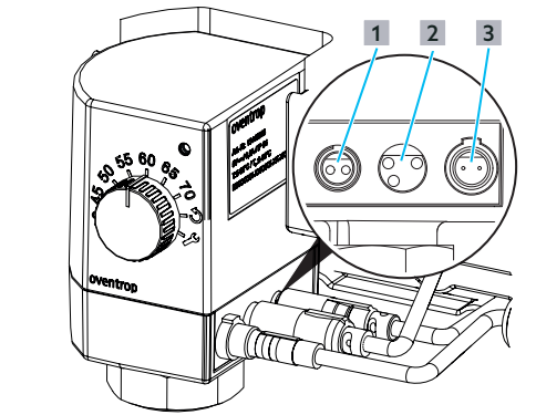
Abb. 5: Steckverbindungen
