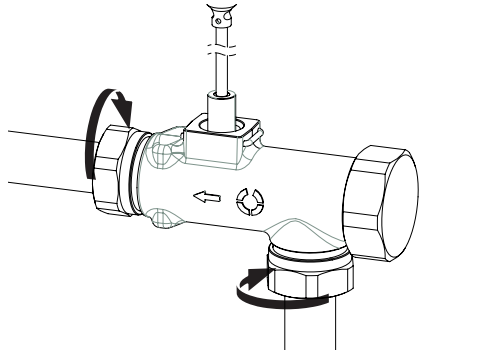
Abb. 4: Volumenstromsensor demontieren
