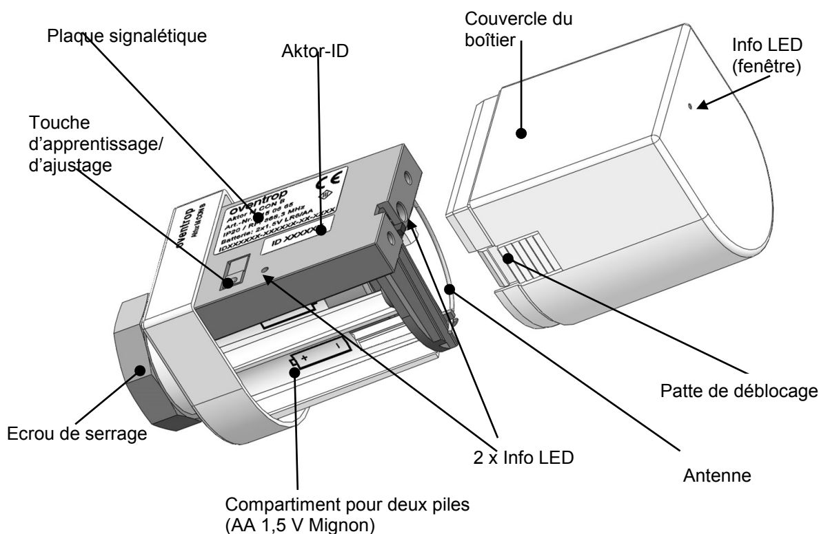
(Fig. 4) Vue intérieure du moteur radio
