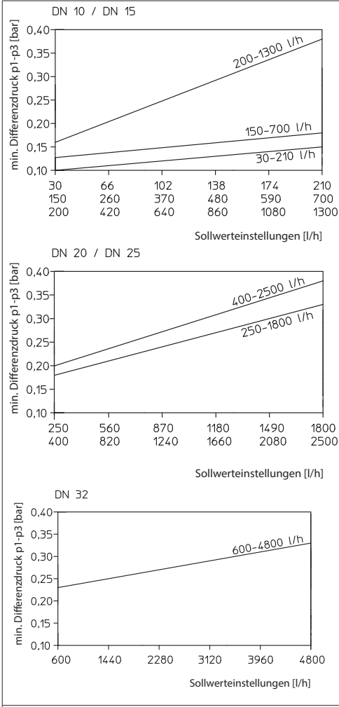
Abb. 13: Mindest-Differenzdrücke
