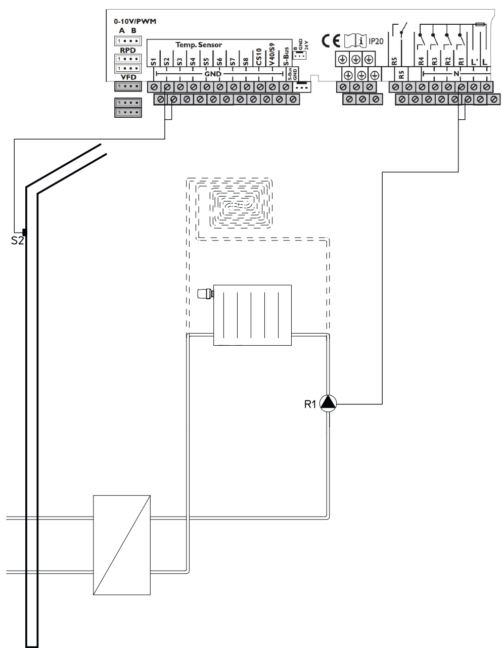
Fig. 52: Schéma 8, un circuit de chauffage direct
