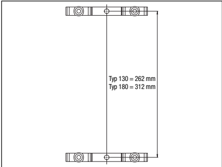
Abb. 6.6 Wandhalterungen befestigen
