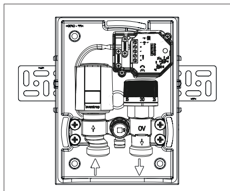
Abb. 9: „Unibox T-RTL R-Tronic“ mit Winkeln
