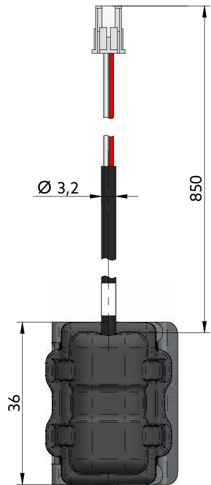
Fig. 2: Encombrements
