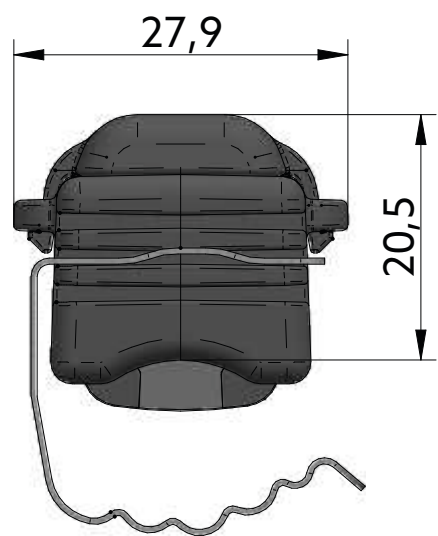
Fig. 3: Encombrements du corps de capteur
