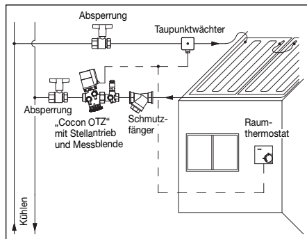
Abb. 6.1 Zweileitersystem
