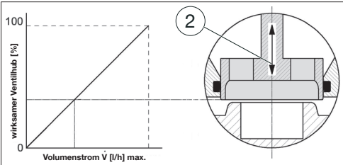
Abb. 5: Lineare Kennlinie der Reguliereinheit
