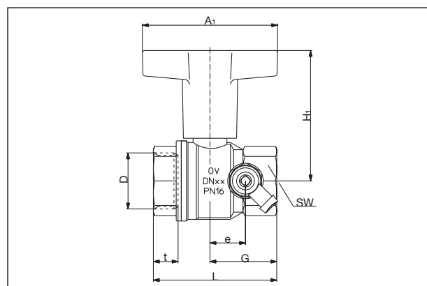
Encombrements réf. 1077804-10 (DN 15 à DN 32) avec manette plastique rallongée
