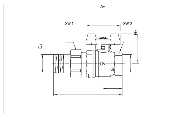
Encombrements réf. 1075804-10 (DN 15 à DN 32) avec manette métallique (DN 15 à DN 25 en aluminium, DN 32 en acier zingué)
