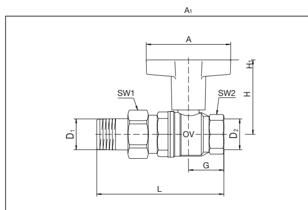
Encombrements réf. 1075704-10 (DN 15 à DN 32) avec manette plastique rallongée
