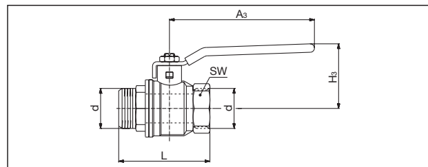
Encombrements réf. 1076203-10 (DN 10 à DN 32) avec levier en acier zingué avec revêtement plastique
