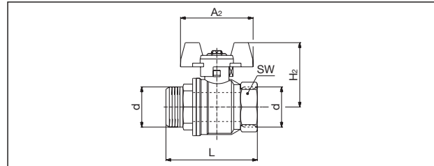
Encombrements réf. 1076303-10 (DN 10 à DN 32) avec manette métallique (DN 10 à DN 25 en aluminium, DN 32 en acier zingué)
