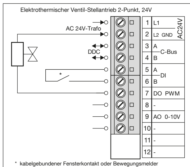
Anschlussbeispiele DynaTemp CR-BX „RBG-C K“
