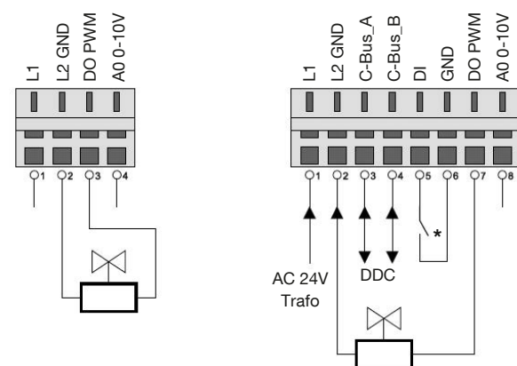
Anschlussbeispiel Raummodule „RM-C F“
