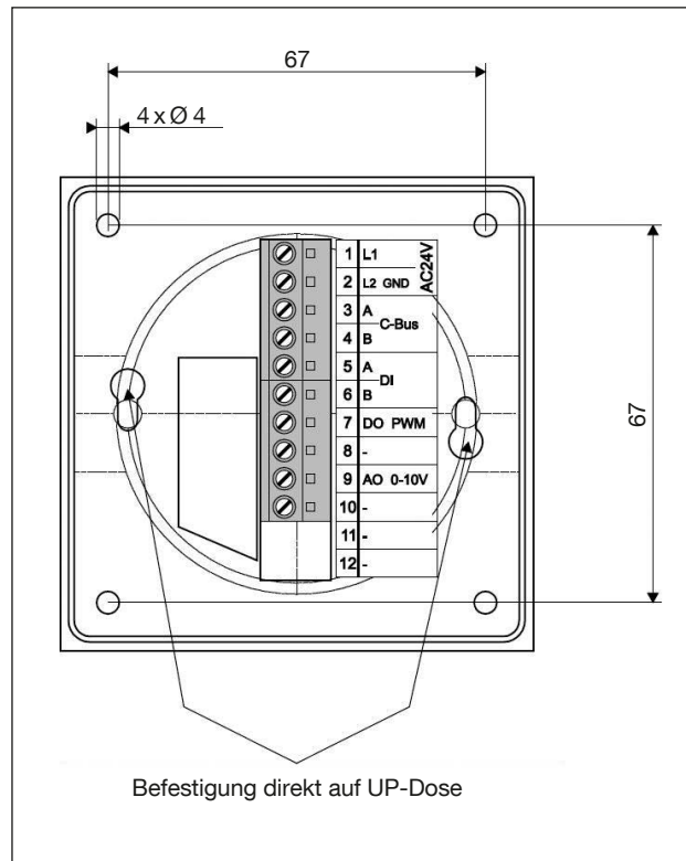
Abmessungen für Bohrungen
