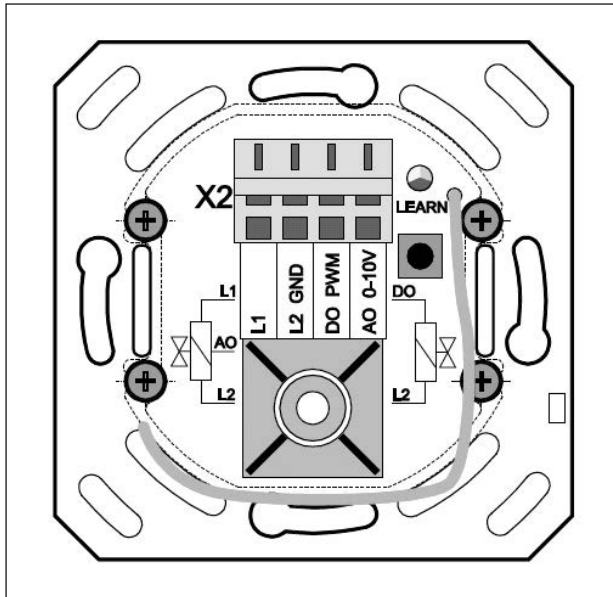
Anschlussbelegung: Frontseitige Anschlüsse
