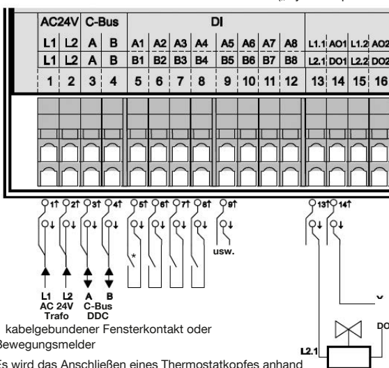
Anschlussbeispiele DynaTemp CR-BX „RM-C F8“
