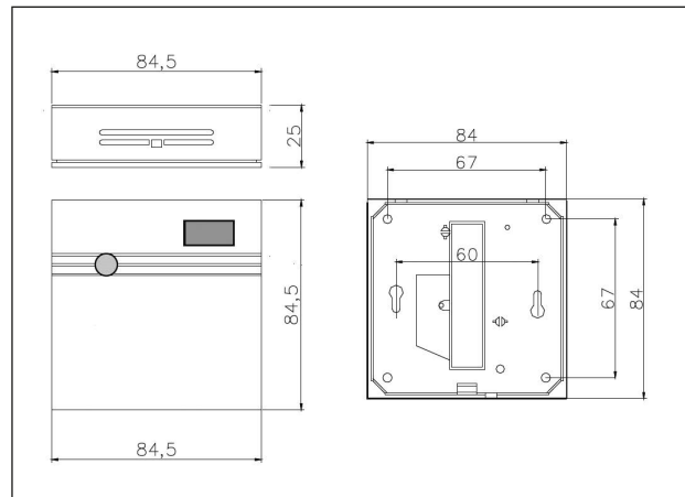
Abmessungen und Maße für Bohrungen
