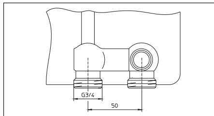
Abb. 9 Ventilgarnitur G \frac{3}{4} AG nach DIN EN 16313 (Eurokonus)
