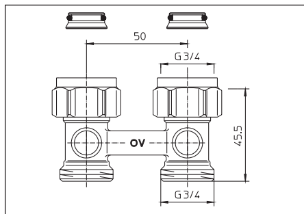
Fig. 4 Modèle droit, G \frac{3}{4} écrou x G \frac{3}{4} mâle
