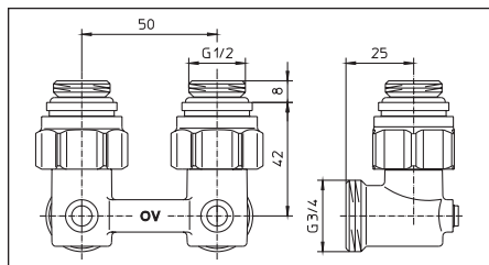
Fig. 7 Modèle équerre, G \frac{1}{2} mâle x G \frac{3}{4} mâle
