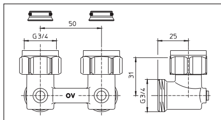
Fig. 6 Modèle équerre, G \frac{3}{4} écrou x G \frac{3}{4} mâle
