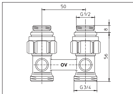
Fig. 5 Modèle droit, G \frac{1}{2} mâle x G \frac{3}{4} mâle
