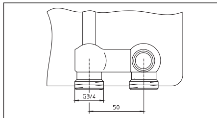
Fig. 9 Robinetterie intégrée G \frac{3}{4} mâle selon DIN EN 16313 («eurocône»)
