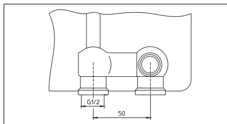
Fig. 8 Robinetterie intégrée G \frac{1}{2} femelle
