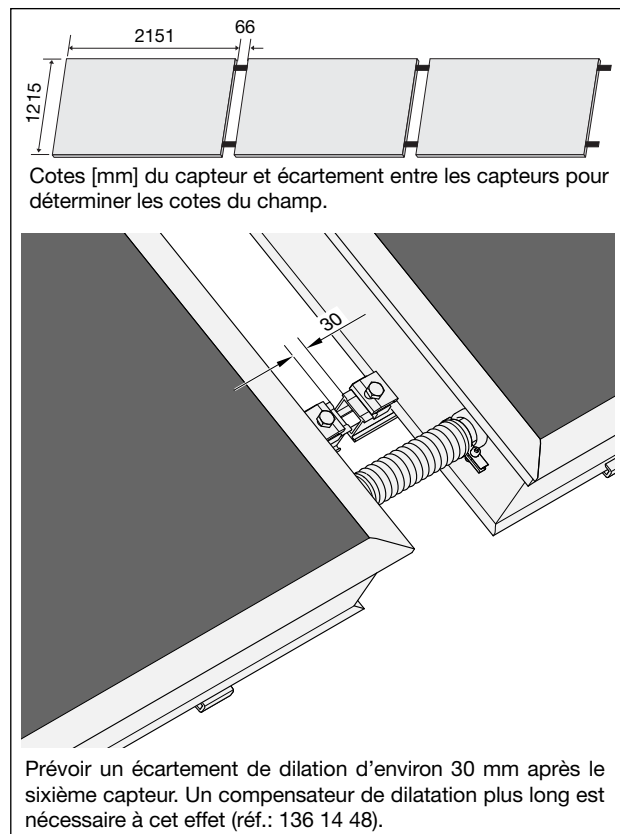
Fig. 8: Écartements entre les capteurs
