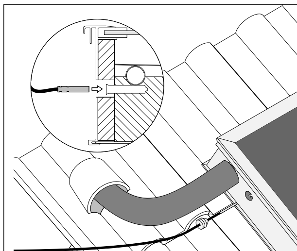
Abb. 37: Fühler durch Gummistopfen ziehen und Fühlerspitze in Fühlerhülse stecken. Gummistopfen wieder eindrehen
