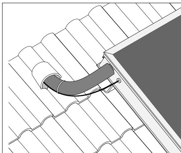
Abb. 38: Fühlerkabel mit Kabelbinder an Anschluss Schlauch befestigen.
