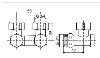
ZB-afsluitkoppeling, haaks 3/4" (3/4" WM x 3/4" BU) Art.nr. 1016212
