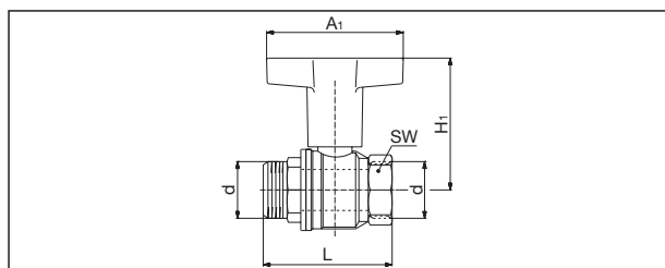
Encombrements réf. 1077303-16 (DN 10 à DN 50) avec manette plastique rallongée
