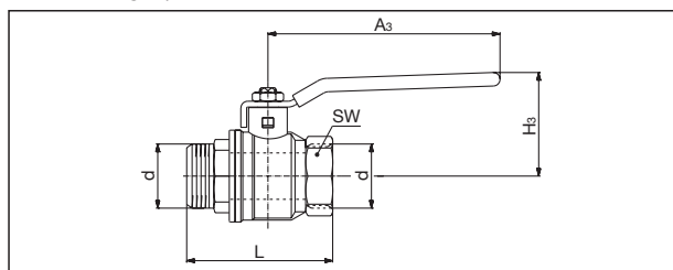
Encombrements réf. 1076203-10 (DN 10 à DN 32) avec levier en acier zingué avec revêtement plastique
