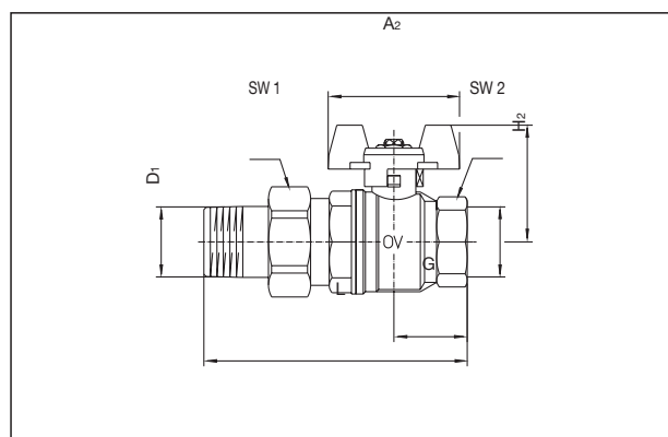
Encombrements réf. 1075804-10 (DN 15 à DN 32) avec manette métallique (DN 15 à DN 25 en aluminium, DN 32 en acier zingué)
