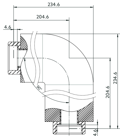
Fig. 5: Encombres du tube coudé
