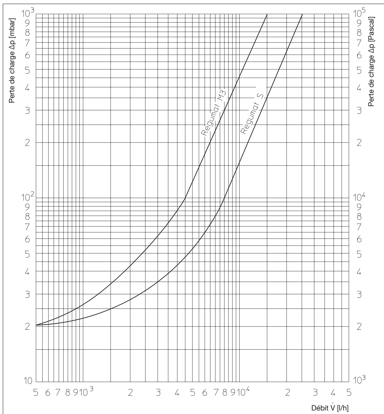
Diagramme de débit
