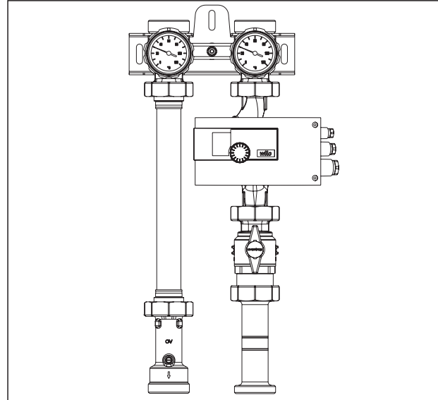
Regumat S-180 plus DN 32 avec robinet d'isolement à tournant sphérique
