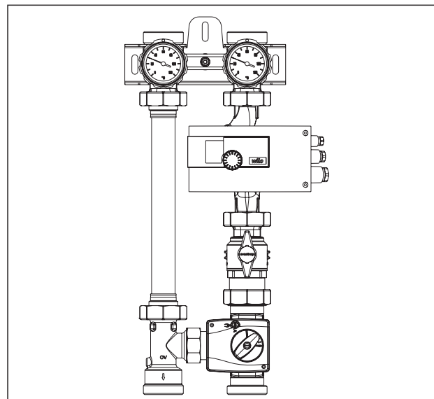
Regumat M3-180 plus DN 32 avec robinet d'isolement à tournant sphérique
