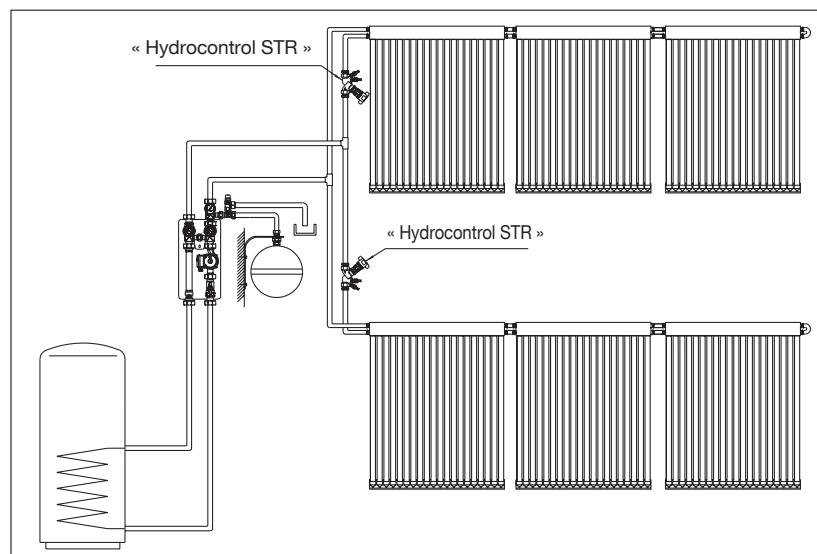
Schéma d'installation
