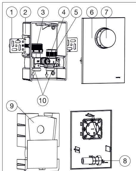
Abb. 2: Aufbau „Unibox T RTL“
