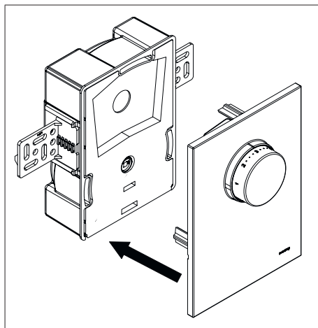
Fig. 11: Pose du capot avec poignée manuelle
