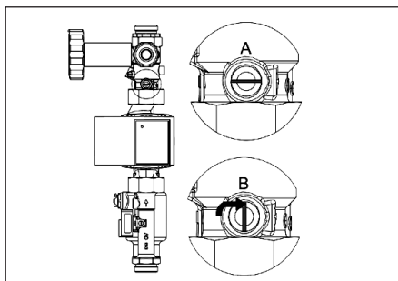
Сх. 6.13 Възвратен вентил (въртящ кран)
