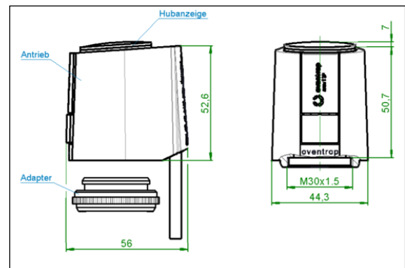
Afmetingen: aandrijving met hulpschakelaar
