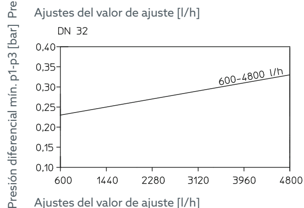
Fig. 13: Presiones diferenciales mínimas
