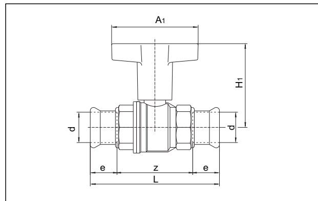
Codice 107 71 62 – 66 (Ø 15 – Ø 35),
