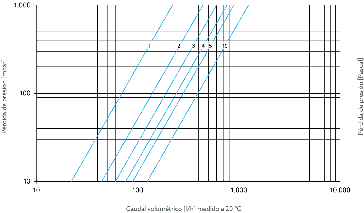
Fig. 15: Caudal volumétrico preestablecido DN 15
