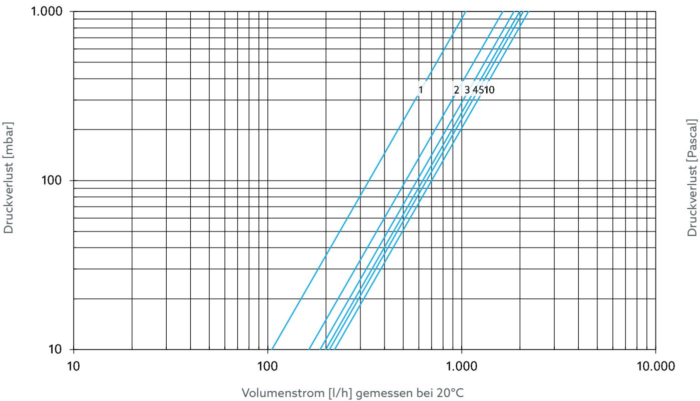
Abb. 16: Volumenstromvoreinstellung DN 20
