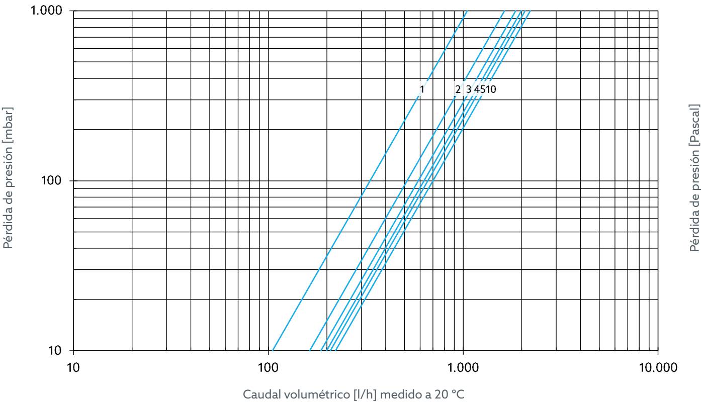
Fig. 16: Caudal volumétrico preestablecido DN 20
