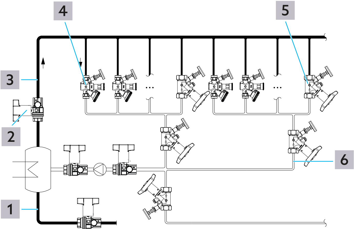
Afb. 4: Installatieschema
