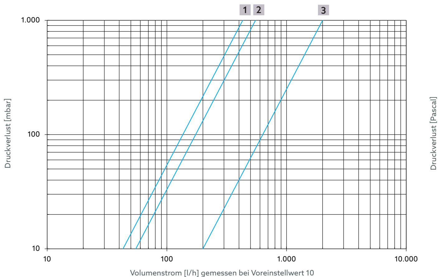
Abb. 20: Volumenstrom Thermische Regelung für Artikelnummer 4202554 und 4202754
