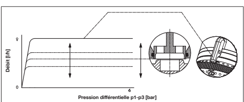
Fig. 4: Pression différentielle p1-p3 (bar)
