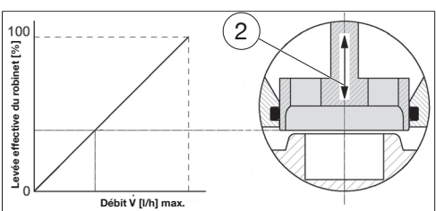
Fig. 5: Courbe de fonctionnement de l'unité de régulation
