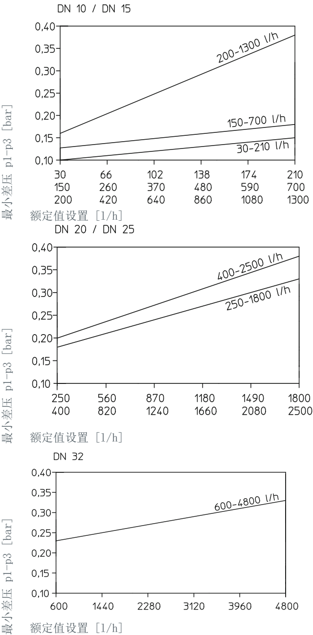
图 13： 最小差压
