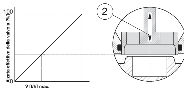
Fig. 5 - Curva caratteristica lineare dell'unità di regolazione
