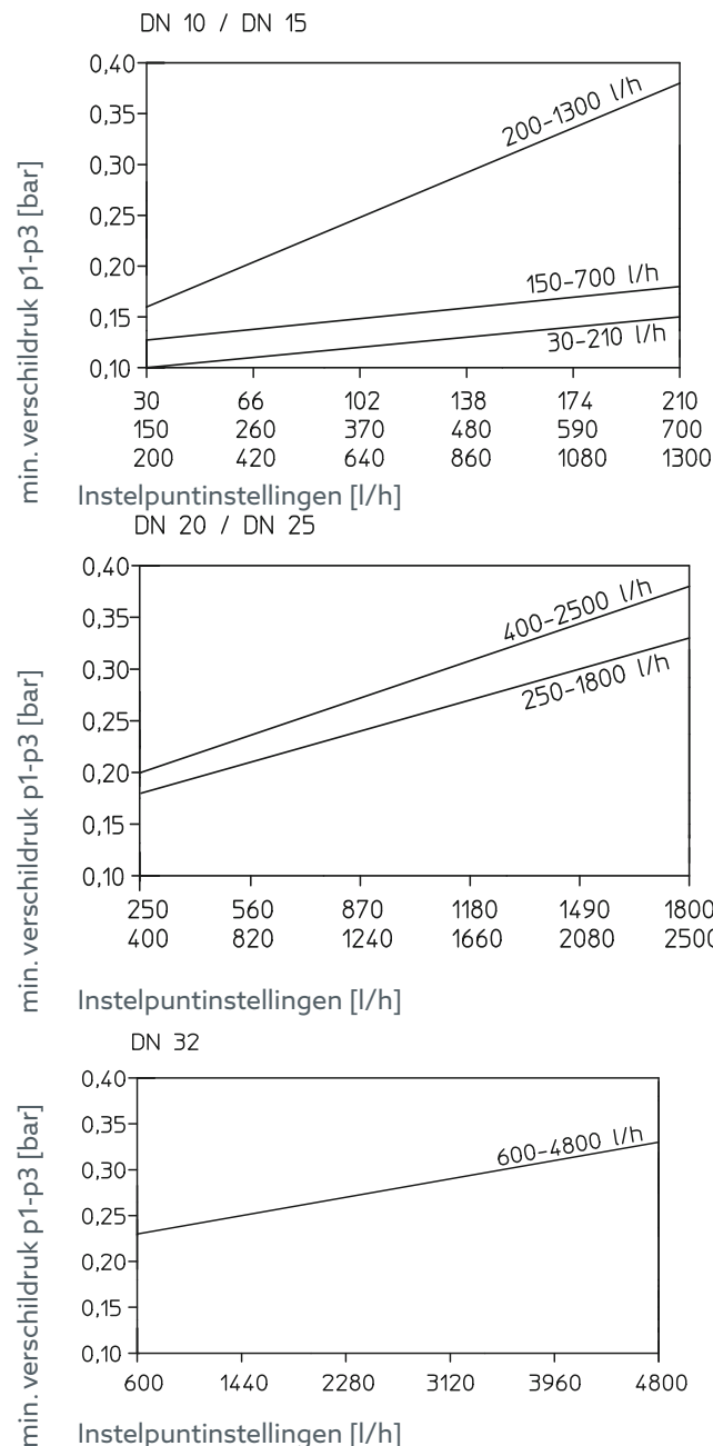
Afb. 13: Minimale verschildrukken
