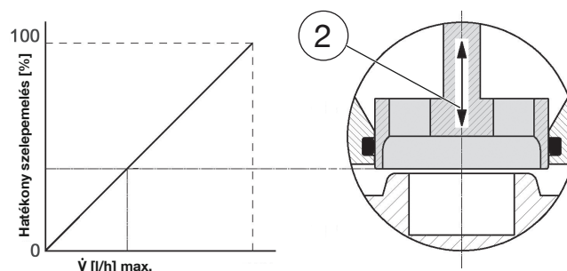
5. A szabályozó egység lineáris funkciós görbéje
