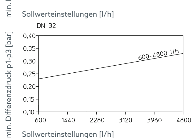
Abb. 13: Mindest-Differenzdrücke
