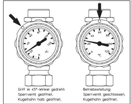
Abb. 30: Kugelhahn
