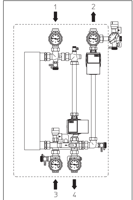
Abb. 19: Versorgungsleitungen anschließen
