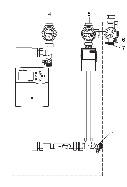
Abb. 29: Primärkreislauf
