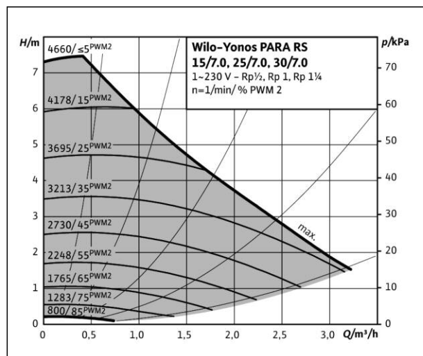
Abb. 5: Pumpenkennlinie Sekundärkreispumpe
