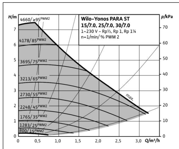
Abb. 6: Pumpenkennlinie Primärkreispumpe
