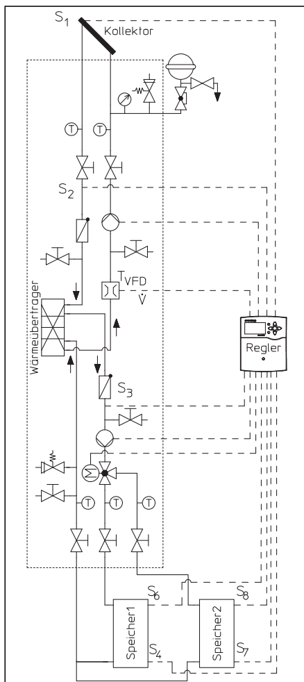
Abb. 25: Ausführung X-Duo Zweispeicherladung
