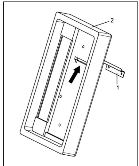
Abb. 17: Unterschale, Wandwinkel
